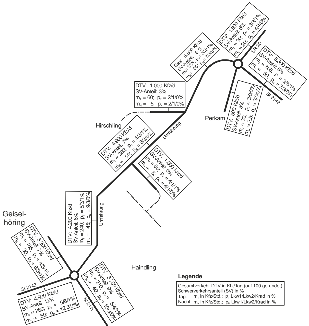
Abb. 4: Kenngrößen für die Lärmberechnungen nach RLS-19 Prognose DTW 2035 mit Umfahrung Geiselhöring, Trasse Haidling-Nord
